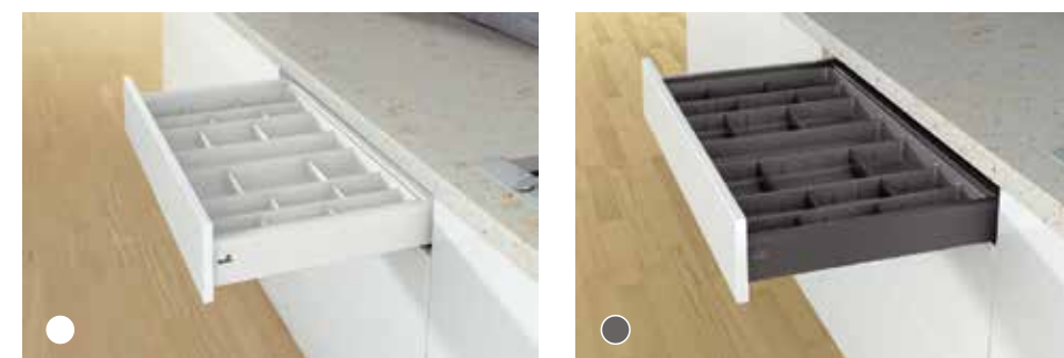
Организационная система OrgaTray 570 Ширина шкафа (номинальная длина направляющих), мм: 600 (500), 900 (500) Пластиковый лоток для приборов с разделительными элементами для индивидуальной организации Для высоты боковины 94мм
